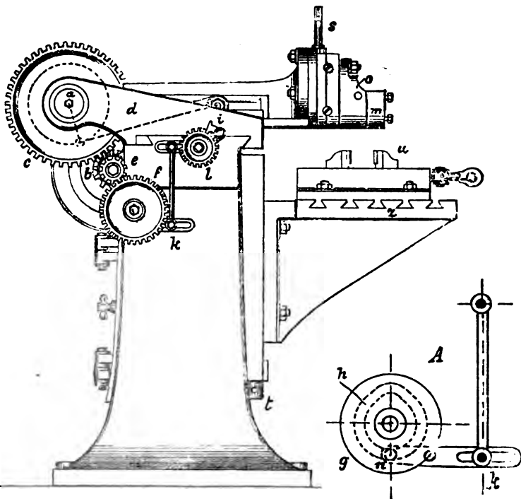
Č 1730. Hoblovací stroj na kovy ( shaping ).
